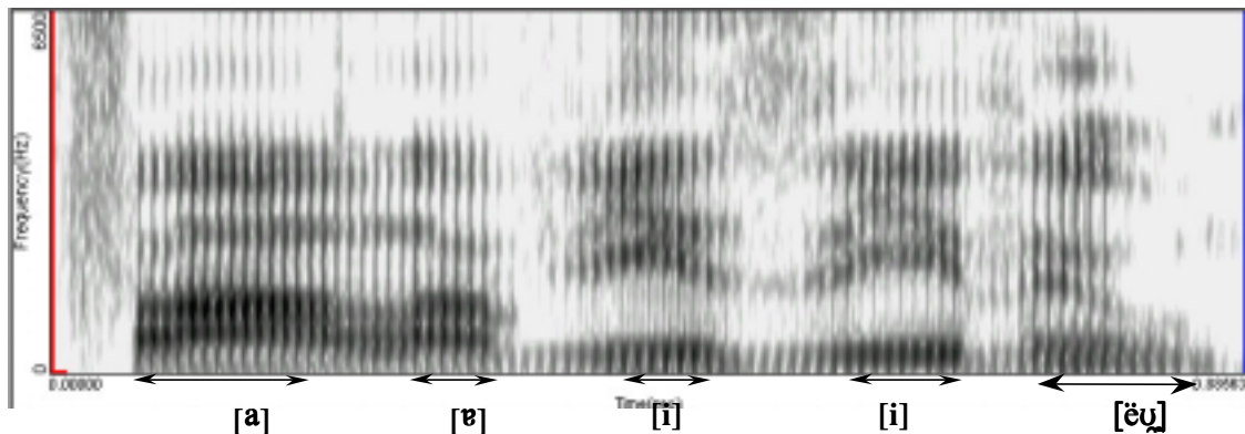
Figura 8: Espectrograma da frase “Fala visível”, produzida pelo Aiuruetê. O enunciado sintético pode ser ouvido em < http://www.lafape.iel.unicamp.br/Docentes/Plinio/plinio_perfil.htm >
