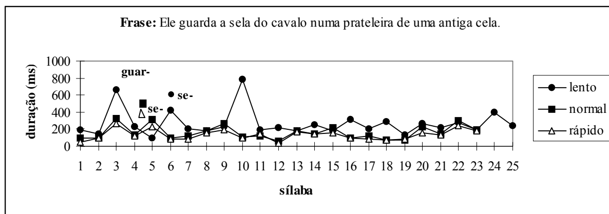
Figura 9: Contornos duracionais para a frase “Ele guarda a sela do cavalo numa prateleira de uma antiga cela.”
