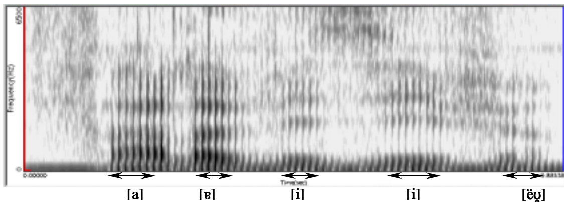
Figura 4: Espectrograma do enunciado “Fala visível”, produzido pelo autor
