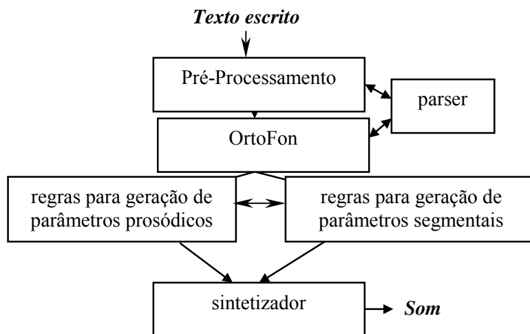
Figura 7: Diagrama geral de um sistema de síntese de fala a partir do texto escrito
